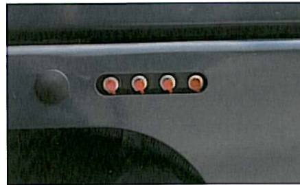
Tuberías de engrase: integrados para un fácil mantenimiento del rodamiento de giro y las botellas
